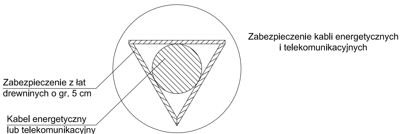
Przekrój A-A
