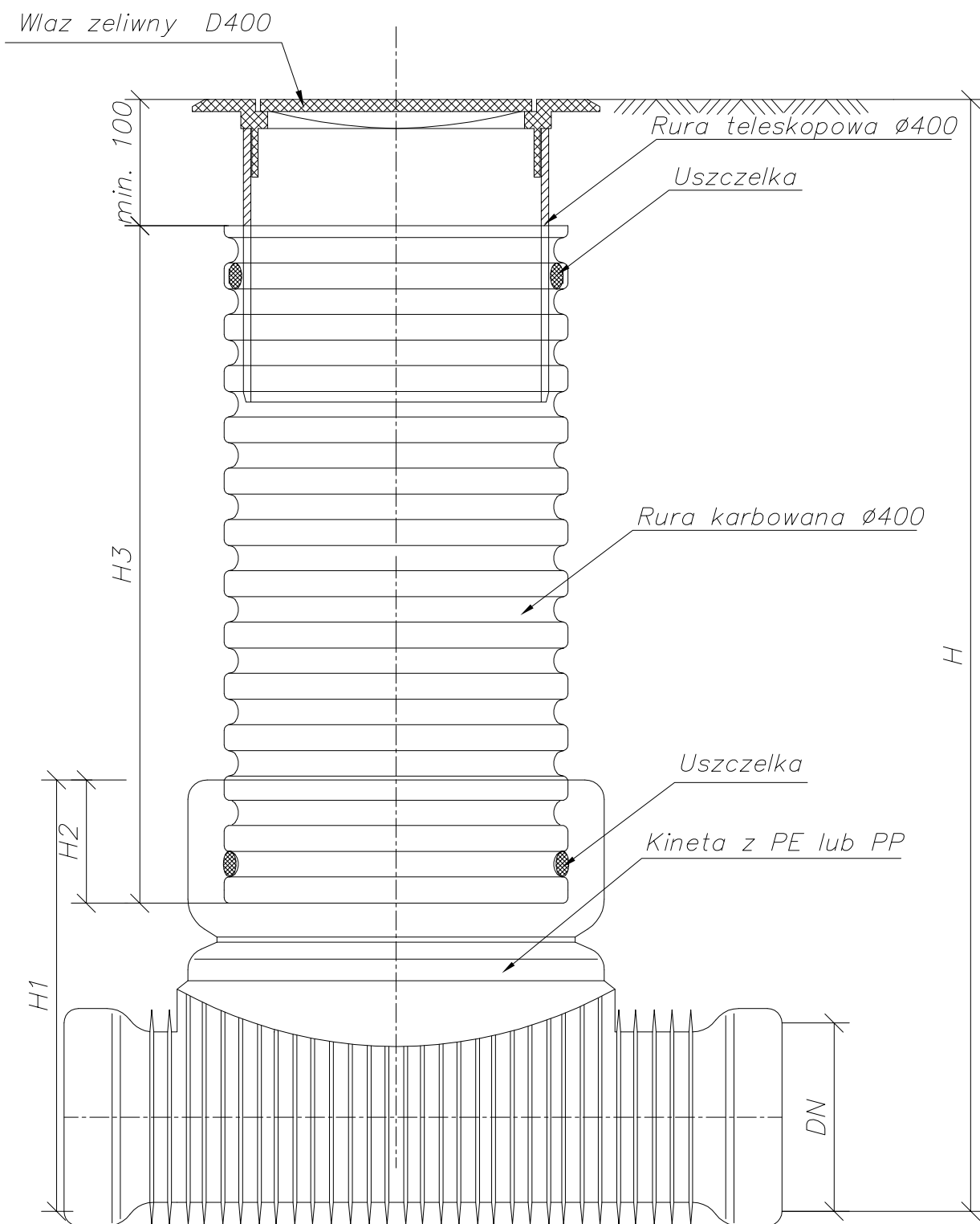
Studzienka kanalizacyjna ø400 niewłazowa
