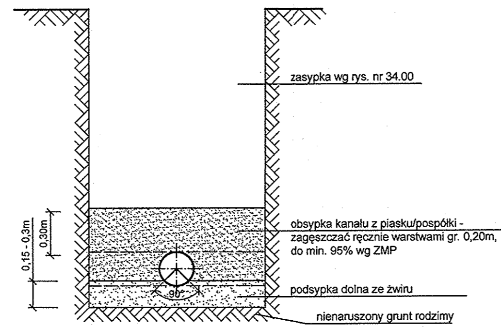
SPOSÓB WYKONANIA STREFY KANAŁOWEJ
