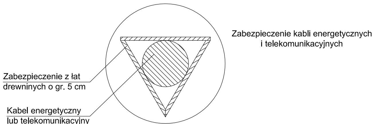
Przekrój A-A
