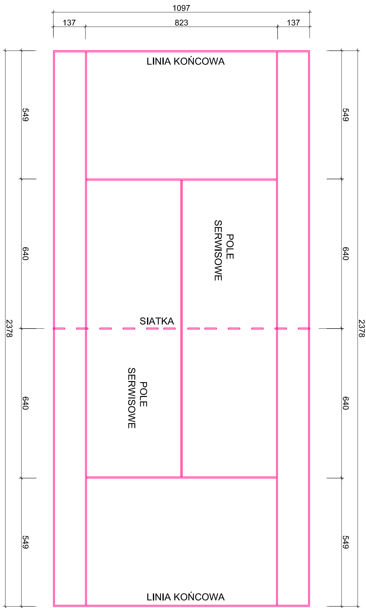
LINIE KORTU TENISOWEGO skala 1:100
