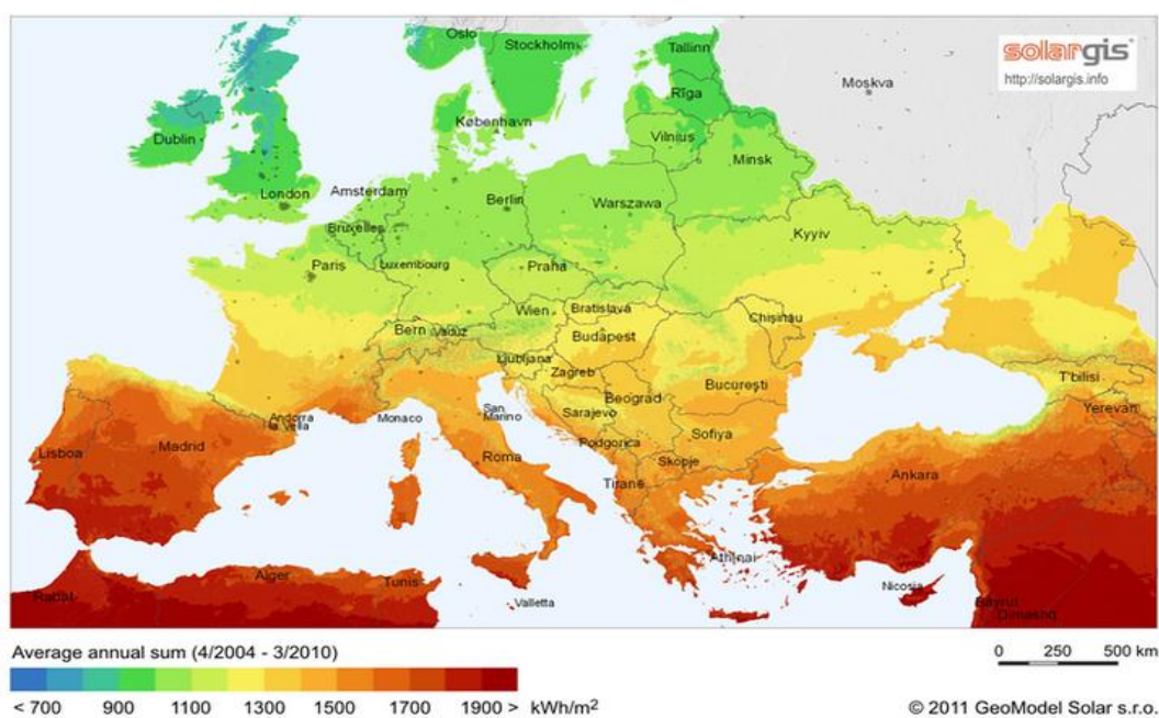
RYSUNEK 30: POTENCJAŁ WYKORZYSTANIA ENERGII SŁONECZNEJ NA TERENIE CAŁEJ EUROPY
