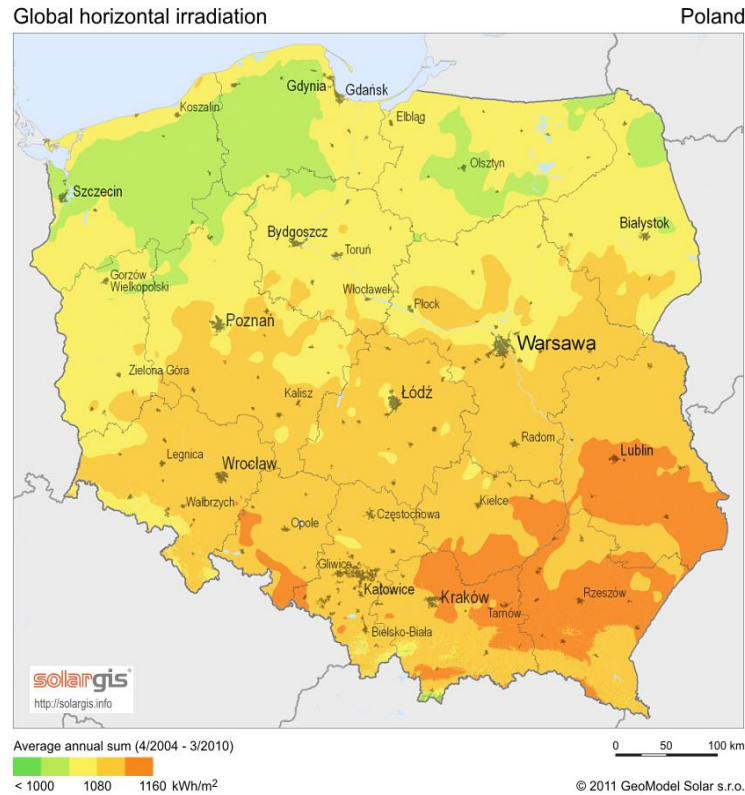
RYSUNEK 31: POTENCJAŁ WYKORZYSTANIA ENERGII SŁONECZNEJ W POLSCE
